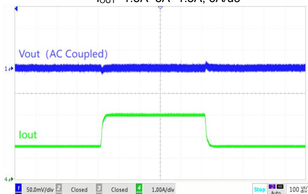
动态负载 I_{OUT}=1.5\text{A}\sim 3\text{A}\sim 1.5\text{A} , 6\text{A}/\mu\text{s}
