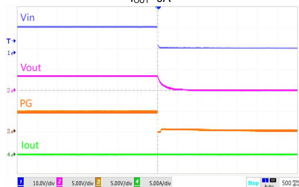
VIN关机 I_{OUT}=0\text{A}
