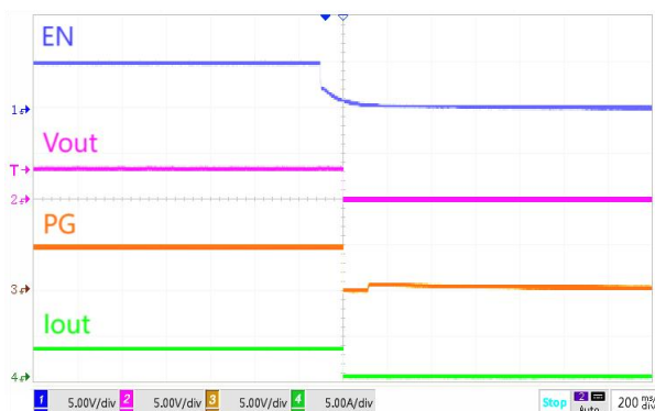
EN关机
