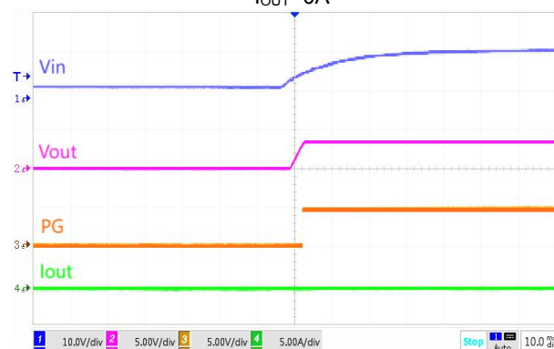
V_{IN} 开机 I_{OUT}=0\text{A}
