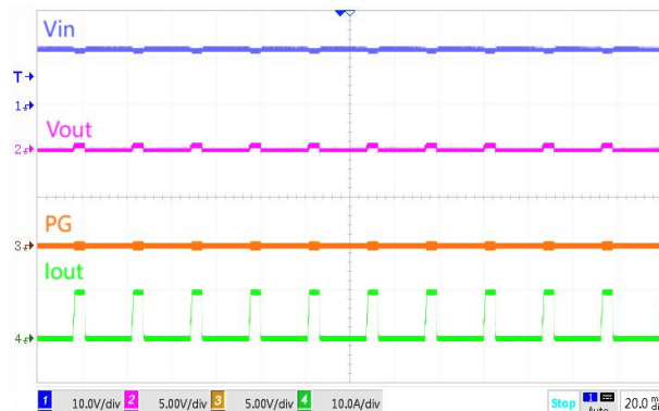
短路 (SCP) 稳态
