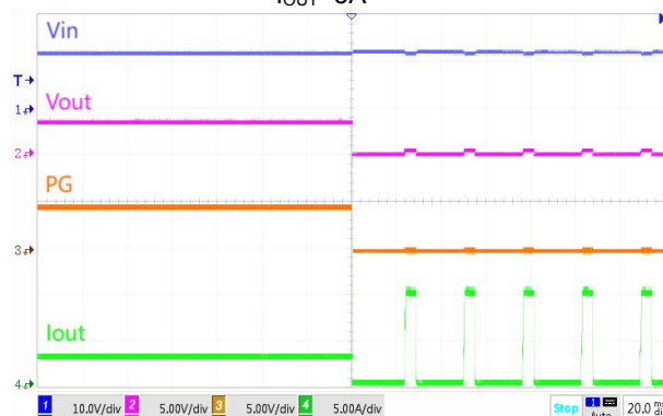
短路保护 (SCP) 进入
