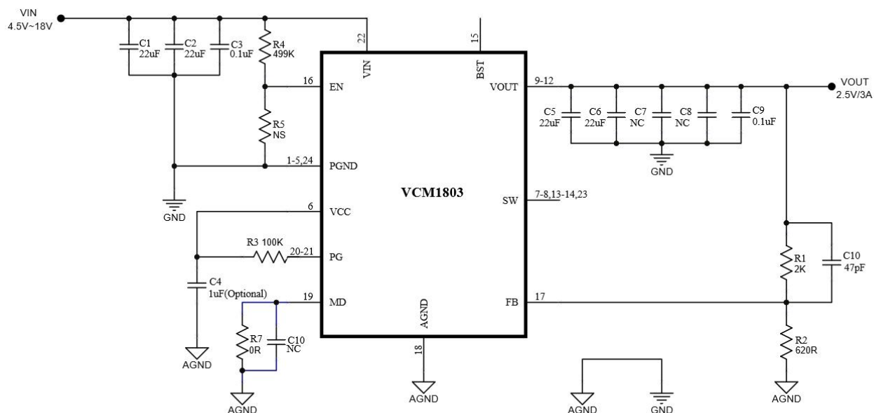
2.5V输出典型应用电路 ( f_{sw}=600kHz , PSM)
